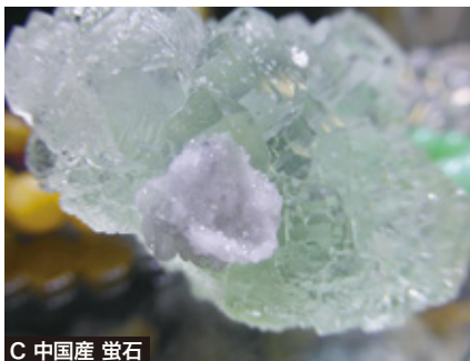
C 中国産 蛍石
