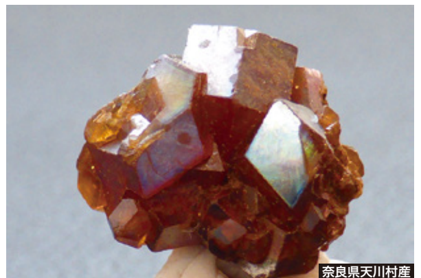
奈良県天川村産
